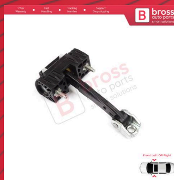
BDP759 Front Door Hinge Stop Check Strap Limiter for Peugeot 407 6E 6D 2004- 2011 4/5 Door 9181J0
